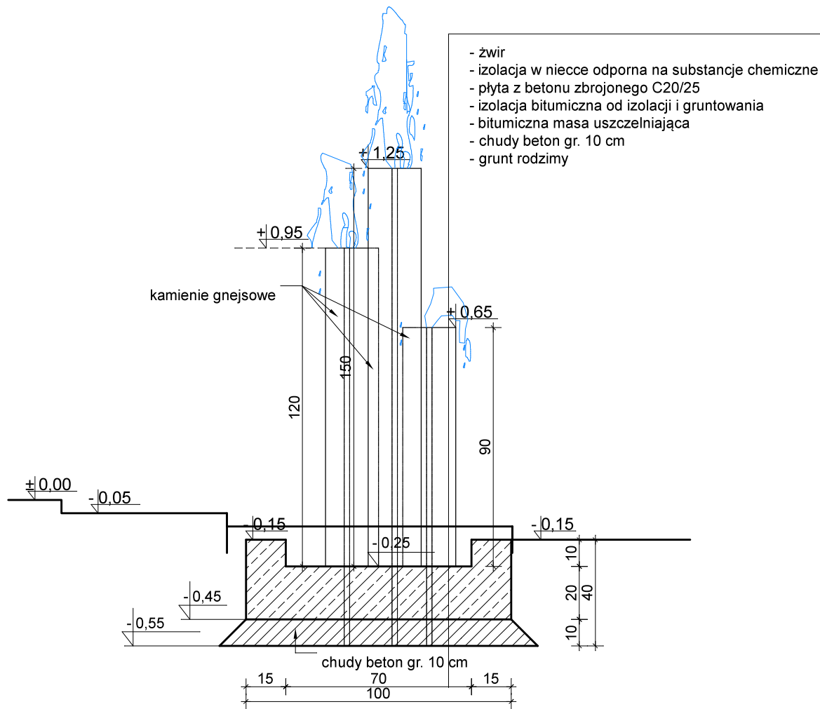
PRZEKRÓJ A-A skala 1:50
