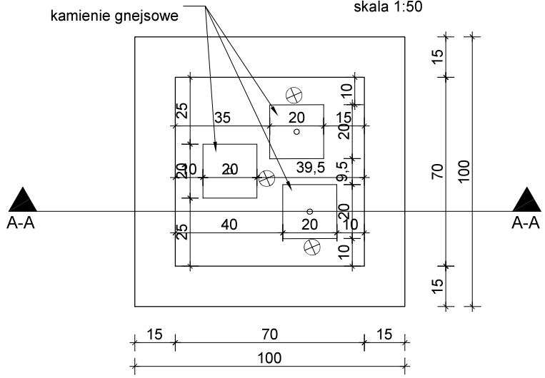
RZUT FONTANNY skala 1:50
