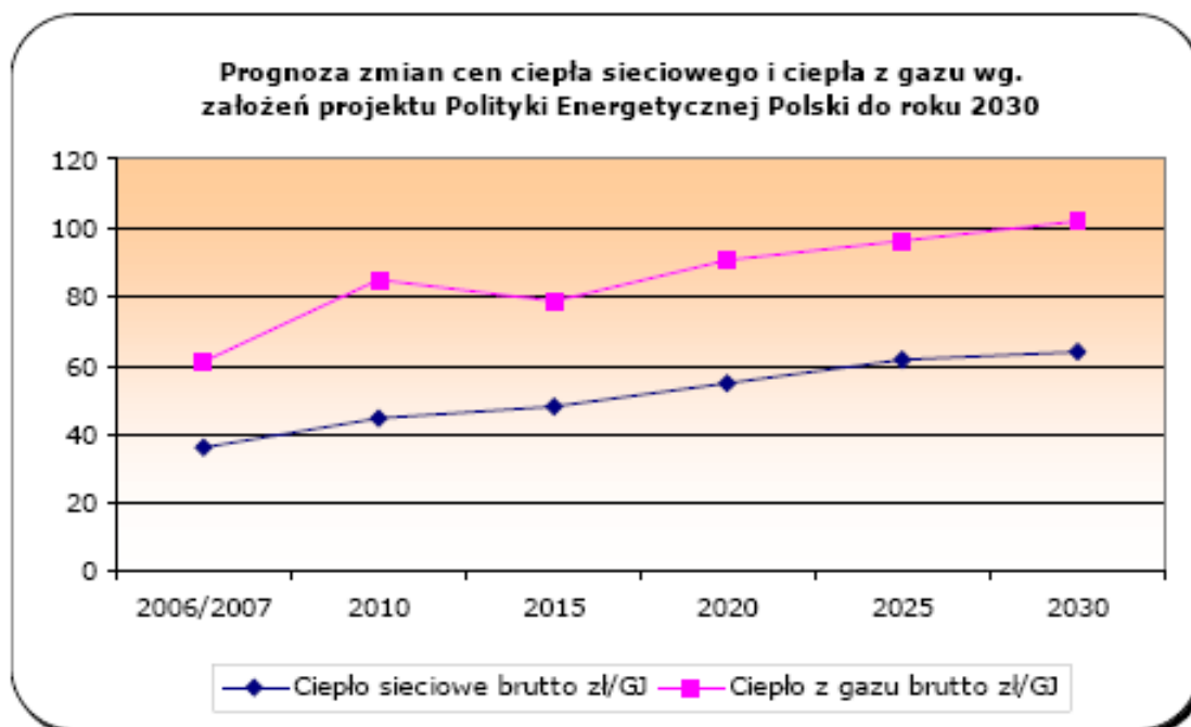
Rysunek 0-26 Prognoza cen ciepła sieciowego i gazowego według Polityki energetycznej Polski do roku 2030. [źródło: Projekt: Uciepłnienie osiedla Żabinek]
