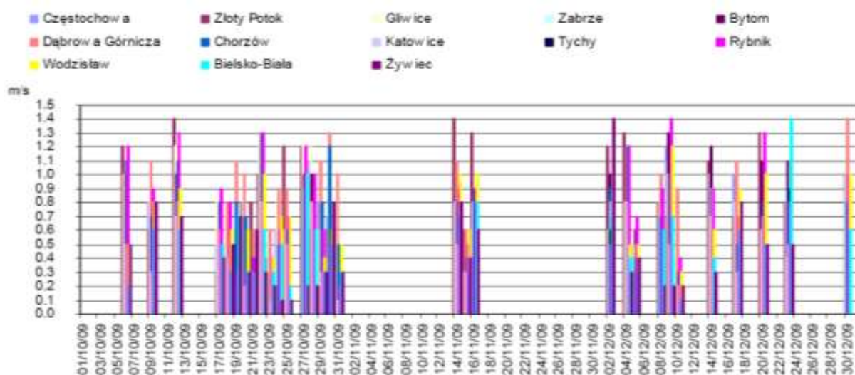
Rysunek 0-16 Okresy występowania niekorzystnych warunków meteorologicznych zanotowane na stacjach automatycznych monitoringu powietrza w od 1.10.2009 r. do 30.12.2009 r. (źródło: Ósma roczna ocena jakości powietrza w województwie śląskim za 2009 r. – WIOŚ Katowice)
