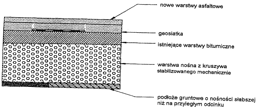
Rys. 2. Wzmocnienie nawierzchni asfaltowej w strefie zmiany nośności podłoża gruntowego
