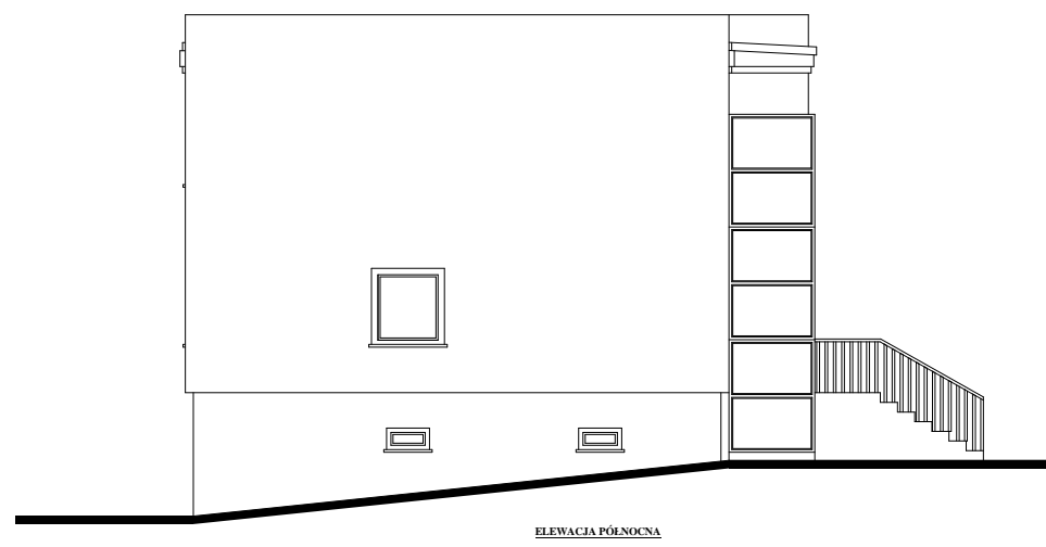
ELEWACJA PÓŁNOCNA
